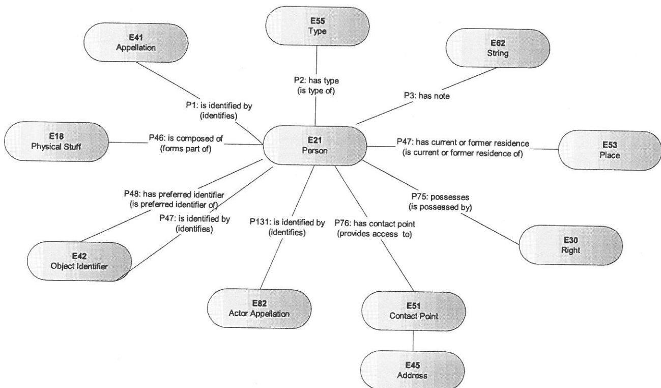
Abb. 3: Einige Beziehungen der Klasse „E21 Person“
