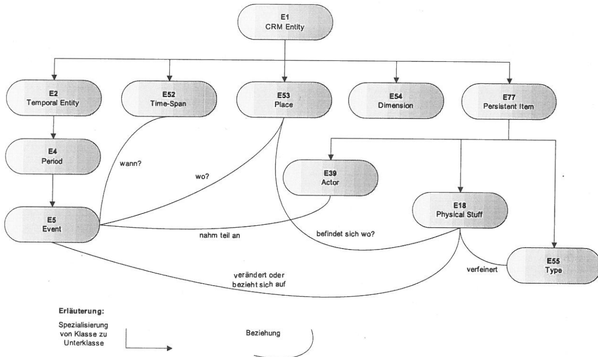
Abb.1: Wichtige Klassen (Entities) der CRM-Klassenhierarchie
